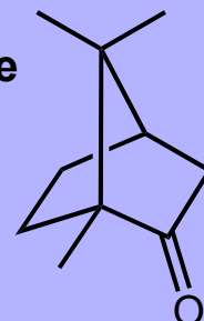
Camphor (Vicks Vap-o-rub)
