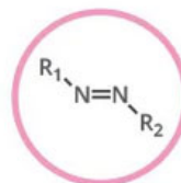
AZO COMPOUND Naming: -azo- e.g. azoethane
